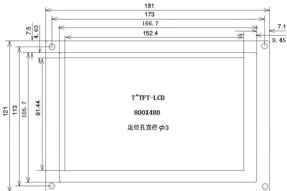
LJD-ZU070尺寸图
